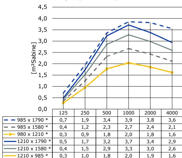
Ekvivalent ljudabsorptionsarea per objekt [m 2 Sabine]
