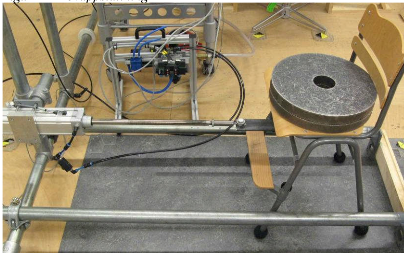
Figur 1 Provpuppställning
